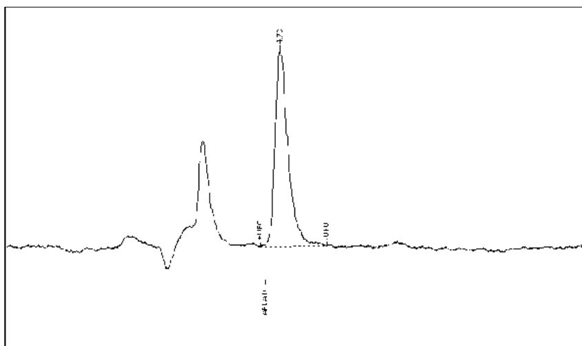
Рис. 1. Хроматограма афлатоксину В1 з концентрацією рівною 0,0165 мг/дм 3 , отримана з використанням флуоресцентного детектору
