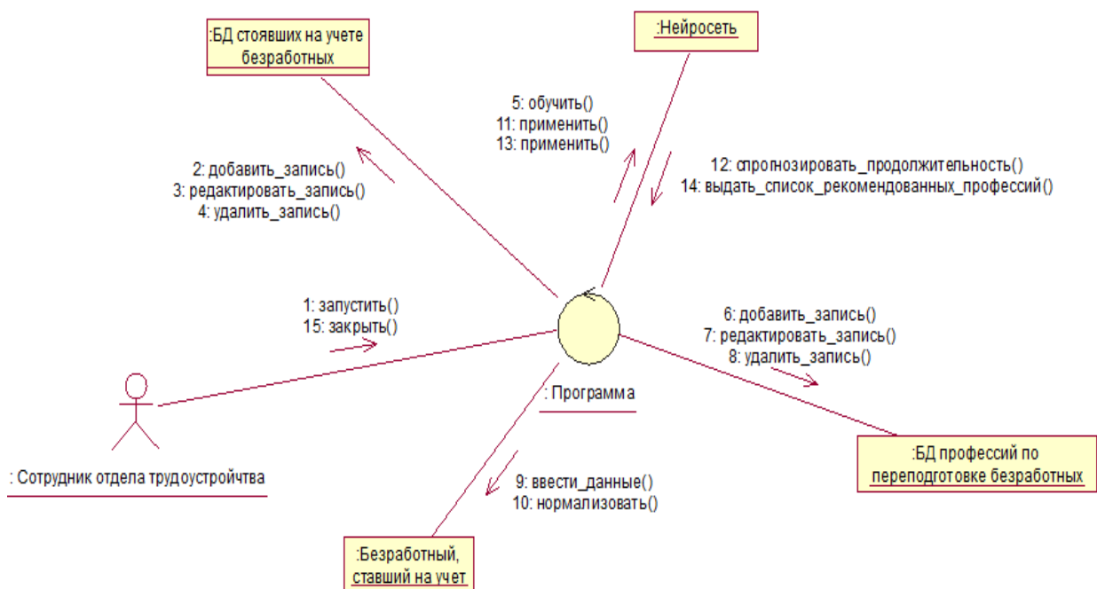
Рисунок 3 – Диаграмма кооперации
