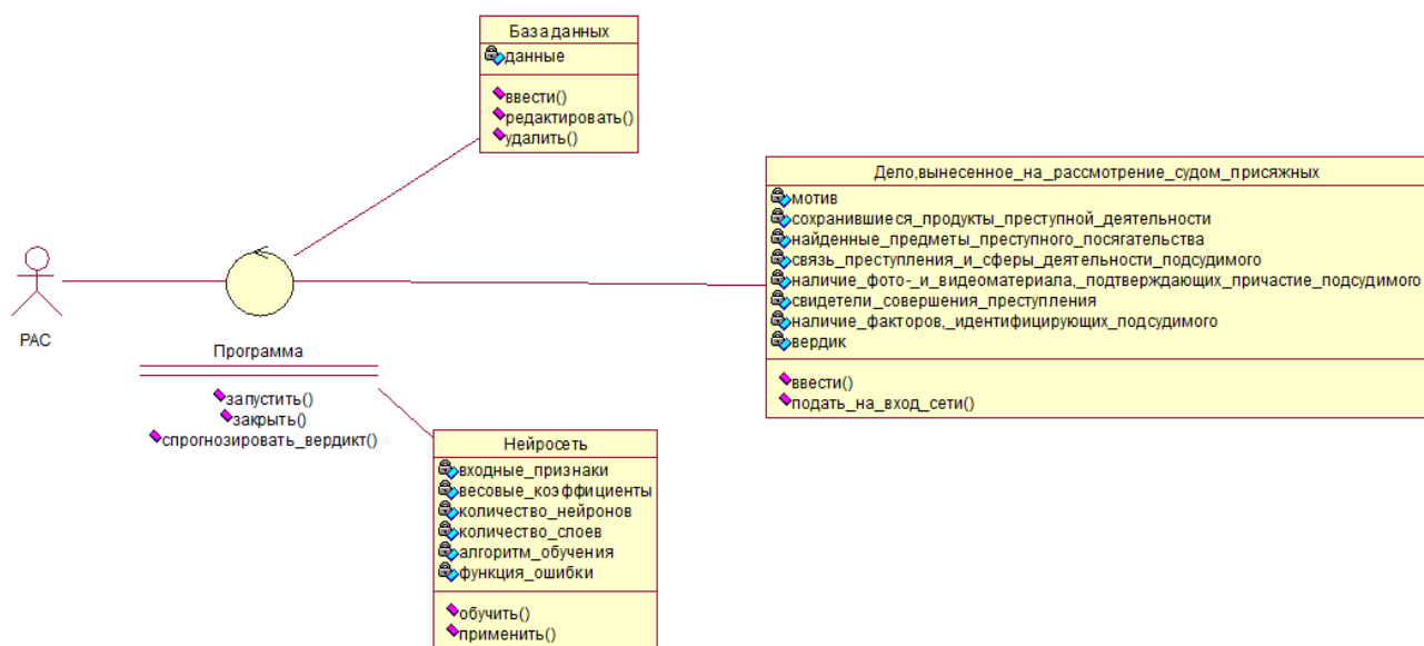
Рисунок 3 – Диаграмма классов
