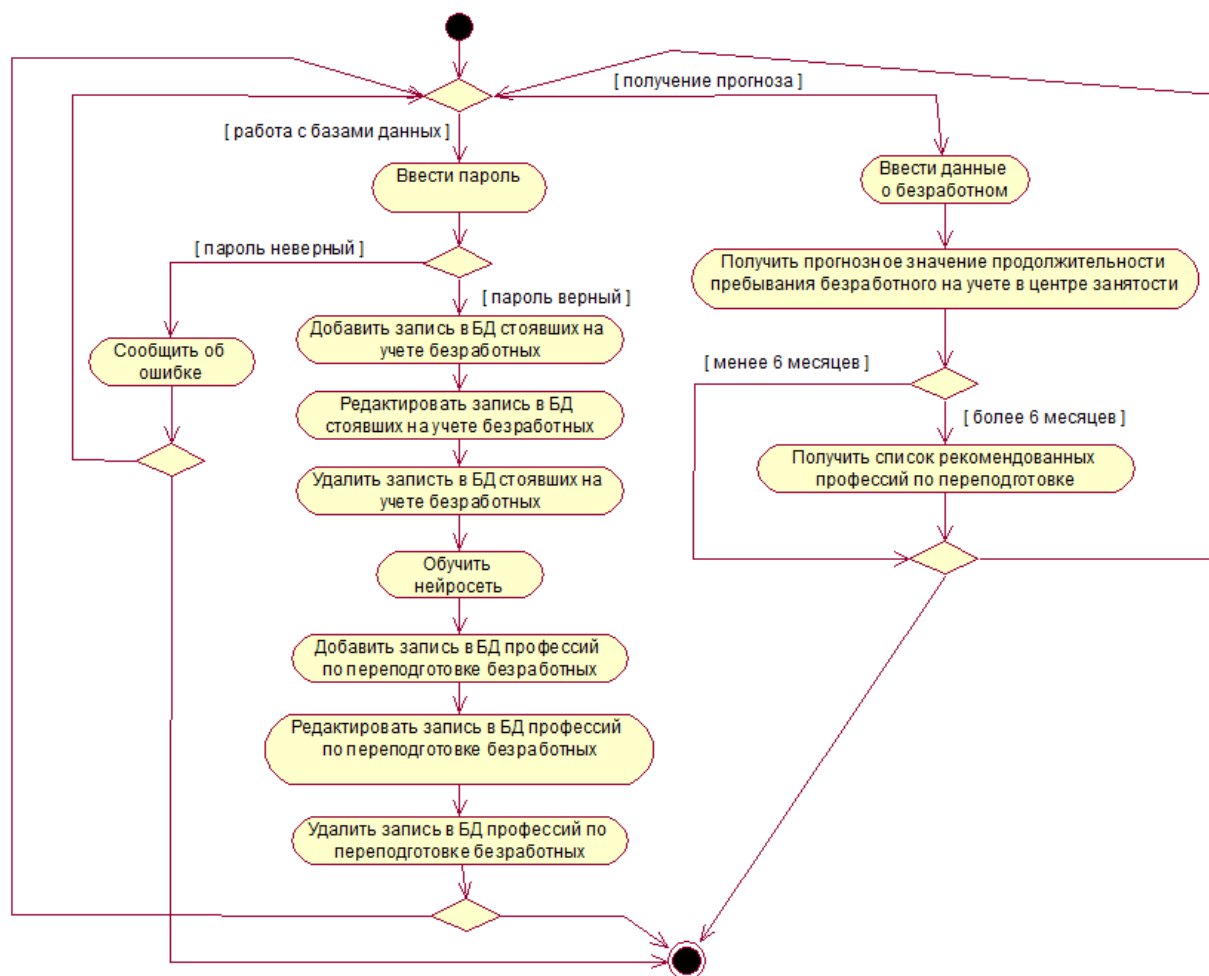
Рисунок 4 – Диаграмма деятельности
