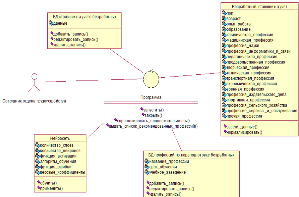
Рисунок 2 – Диаграмма классов
